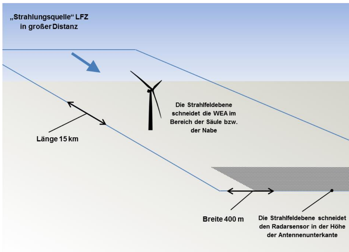
Abbildung 4: Anordnung von Radar und WEA sowie Lage des in dieser Untersuchung dargestellten Luftraums mit einer Ausdehnung von (hier) 15 km x 400 m Breite. Das LFZ wird in einer Distanz von bis zu 130 NM angenommen. – schematische Darstellung –
