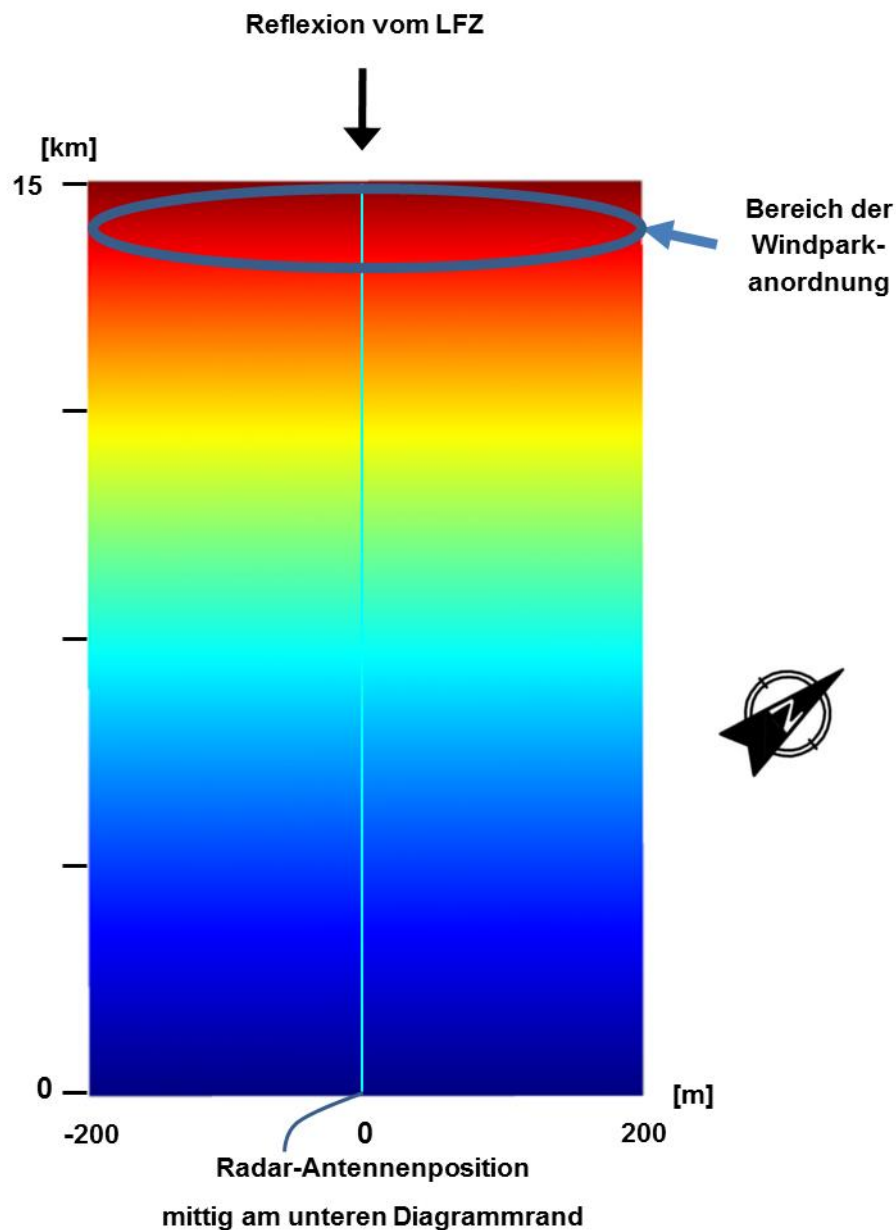
Abbildung 5: Feldgebiet von 15 km x 400 m in der Übersicht (schematische Übersicht für das Radar Brockzetel)
