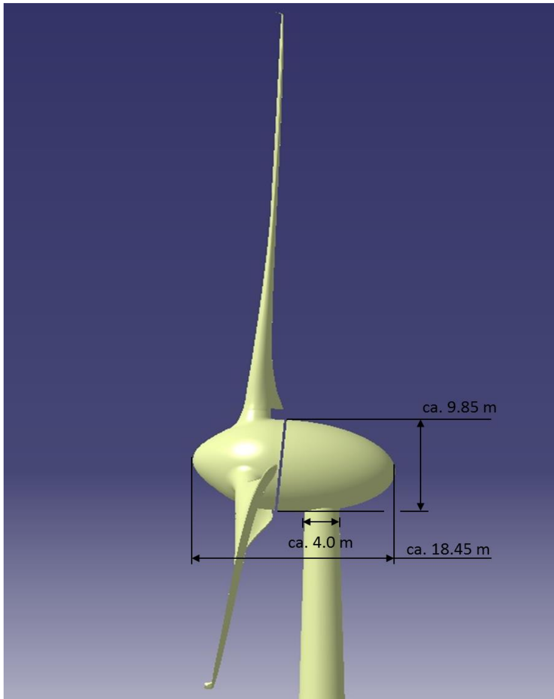
Abbildung 2: Schematische Objektgeometrie für die geplante WEA-Bauform Enercon E126-EP4 ohne Getriebe mit ca. 127 m Rotor bei ca. 135 m NH.
