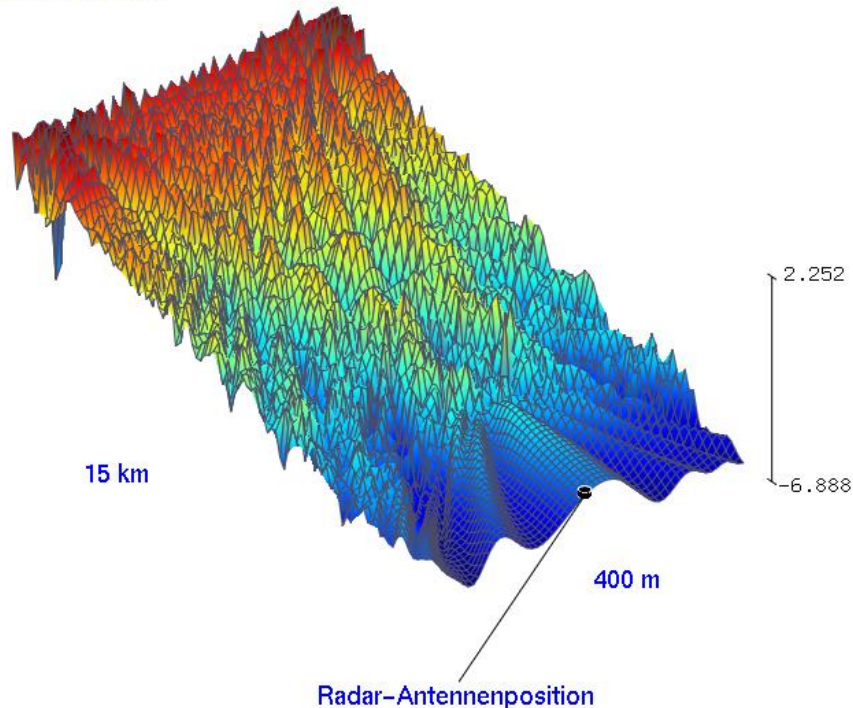
Abbildung 7: Reflexions- und Streufeldausbildung für die Windenergieanlagen an den Standorten WEA 1, WEA 21, WEA 25, WEA 20 und WEA 2 als Fünffach-Anordnung im Einflussbereich der Radaranlage Brockzetel.
