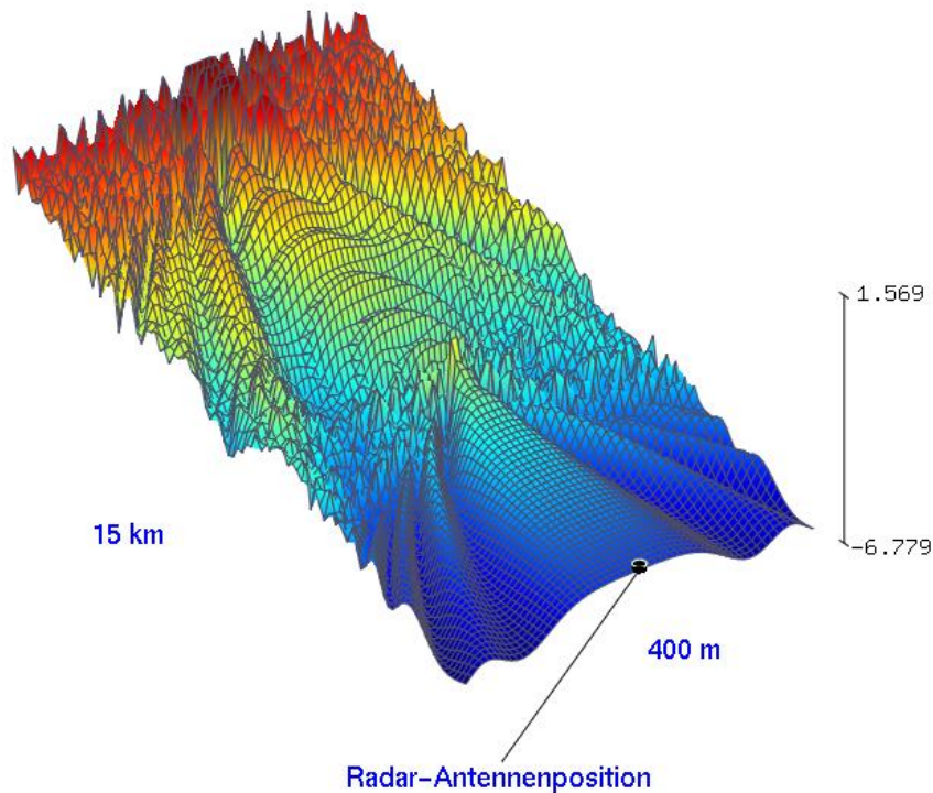
Abbildung 8: Reflexions- und Streufeldausbildung für die Windenergieanlagen an den Standorten WEA 24, WEA 3, WEA 2 und WEA N3 als Vierfach-Anordnung im Einflussbereich der Radaranlage Brockzetel.
